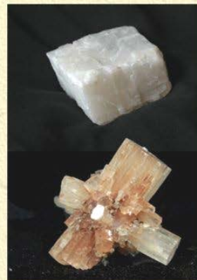
CaCO 3 (Calcita y aragonito)
